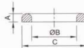
DIN Seal Ring
