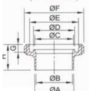
DIN Imperial Welding Male
