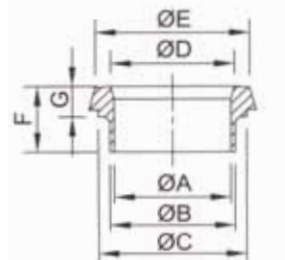
DIN Imperial Welding Liner
