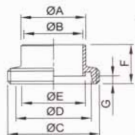
DIN Welding Male DIN-15
