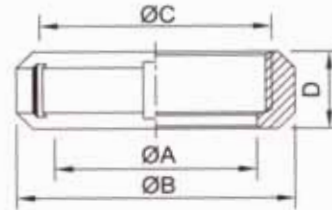
SMS Nut 6 Slots SMS-13R
