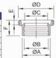
DIN Expanding Male DIN-15R
