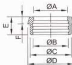
DIN Expanding Liner DIN-14R
